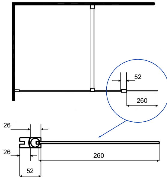
Schemat panelu Eco-N w zakresie 180°
