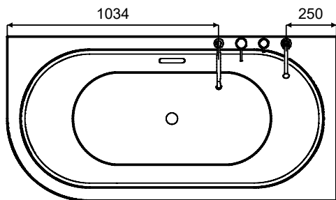
schemat 2/A
