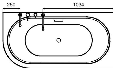
schemat 3/B
