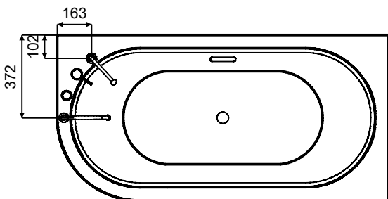
schemat 4/A
