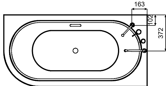
schemat 5/B
