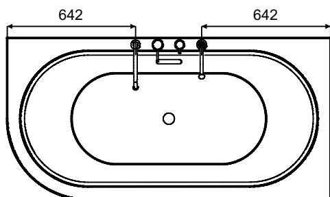
schemat 1/A
