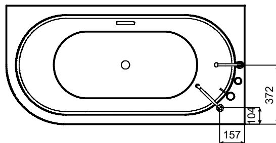
schemat 6/B
